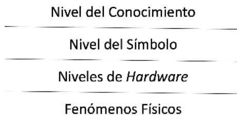
Figura 8.1: Niveles de sistema propuestos por Newell
