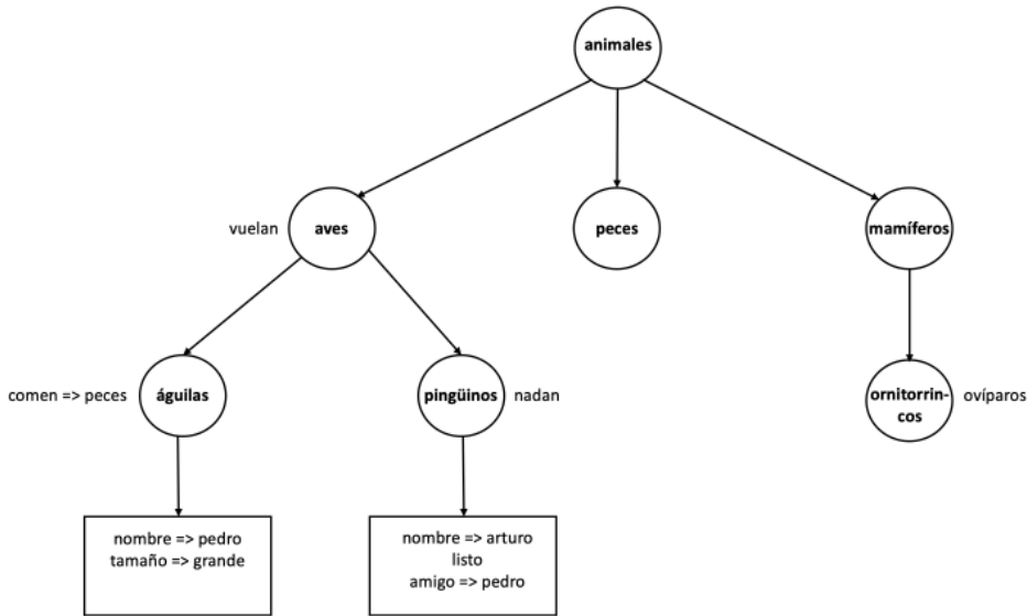
Figura 4.2: Taxonomía de los animales
