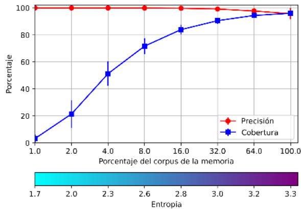
Figura 7.5: Resultados del Experimento 3
