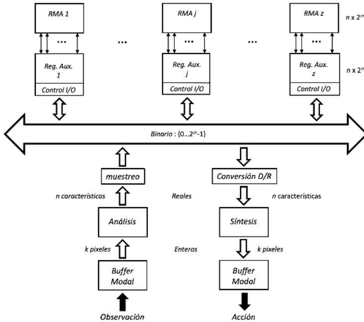
Figura 7.1: Arquitectura de la memoria asociativa
