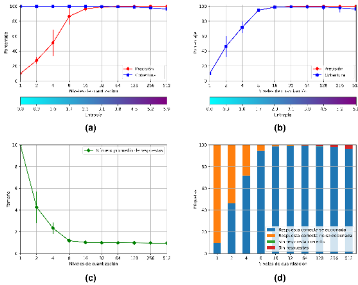
Figura 7.3: Resultados del Experimento 1
