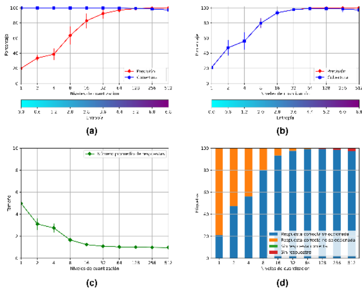
Figura 7.4: Resultados del Experimento 2
