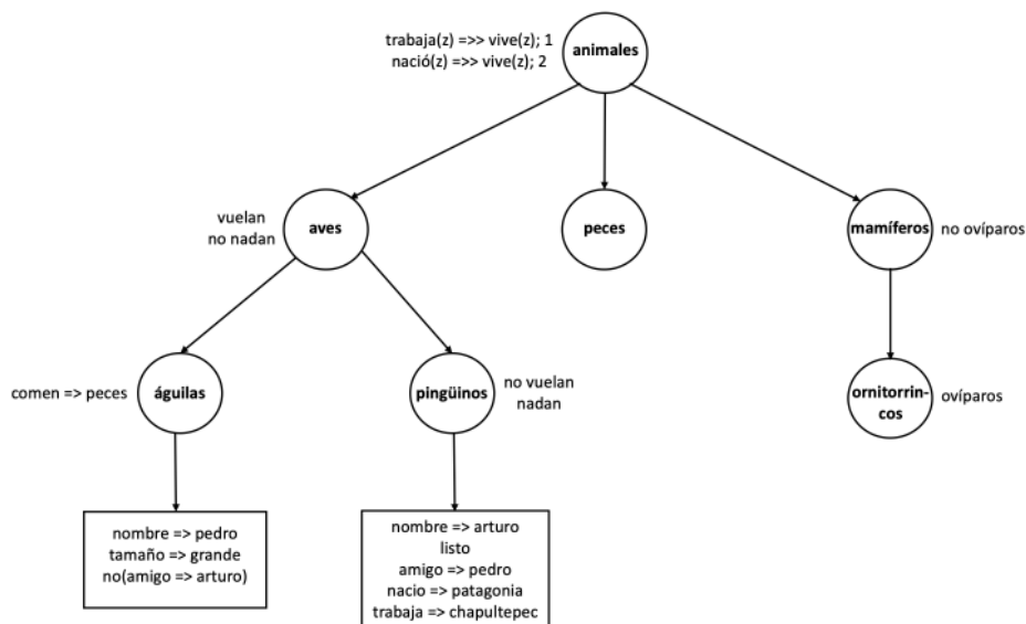
Figura 4.4: Preferencias y Justificaciones
