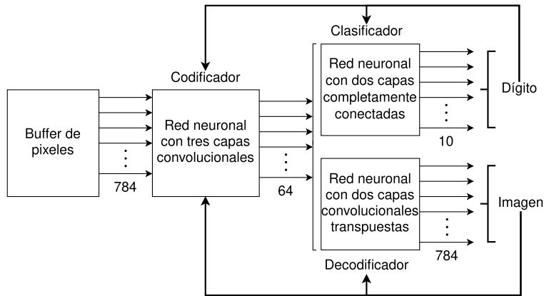
Figura 7.2: Entrenamiento del módulo de análisis
