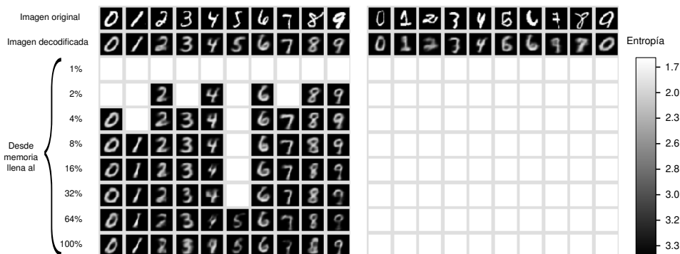
Figura 7.7: Recuperación de memoria con rechazo
