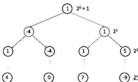
Figura 3.2: Complejidad del Ajedrez
