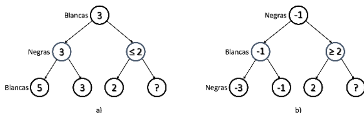
Figura 3.3: Recorte alfa-beta
