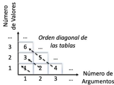
Figura 6.5: Orden de Tablas para Funciones con Dominios y Codominios Finitos
