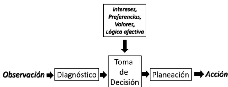
Figura 3.6: Cadena Inferencial
