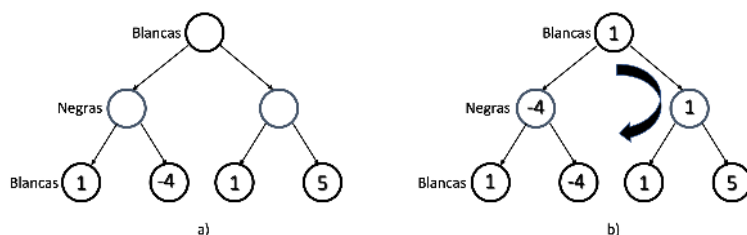
Figura 3.1: Algoritmo Minimax
